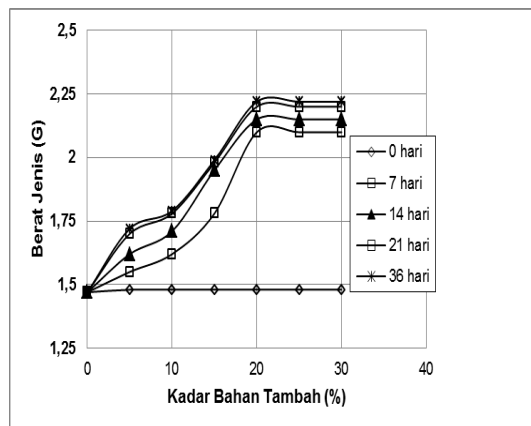
Gambar 4. Hubungan antara Berat jenis-kadar bahan tambah-waktu pemeraman (w = 598%)
