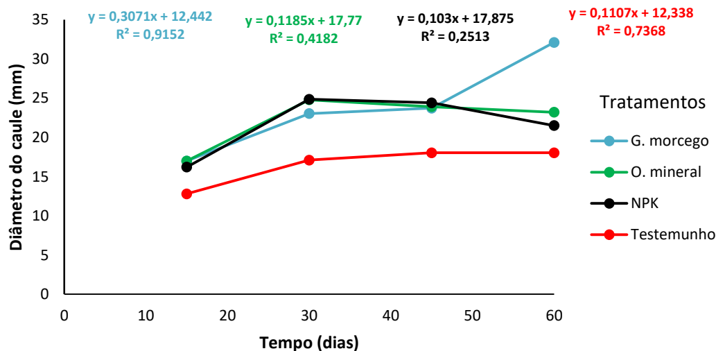
Gráfico 2. Diâmetro do caule (mm) em função da aplicação de fertilizantes orgânicos, minerais e organominerais representado ao longo de 60 dias na cultura do milho. NPK: adubo mineral (12-24-12); G. morcego: adubo orgânico (guano de morcego); O. mineral: adubo organomineral (NPK + guano de morcego); Testemunho (plantas isentas de adubação).
