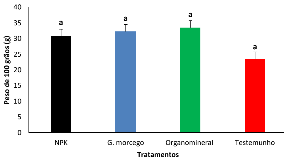
Gráfico 7. Peso de 100 grãos, em função da aplicação de fertilizantes orgânicos, minerais e organominerais. NPK: adubo mineral (12-24-12); G. morcego: adubo orgânico (guano de morcego); Organomineral: adubo organomineral (NPK + guano de morcego); Testemunho (plantas isentas de adubação). As barras de erro representam o erro padrão. Barras com letras iguais não apresentam diferenças significativas no teste de Duncan ( P > 0.05 ).
