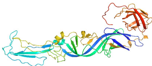
Figura 4. Glicoproteína E1 del virus del chikunguña. Fuente: tomada y adaptada de Protein Data Bank y Fox et al. Cell. 2015; 163(5):1095-107. (47,48).
