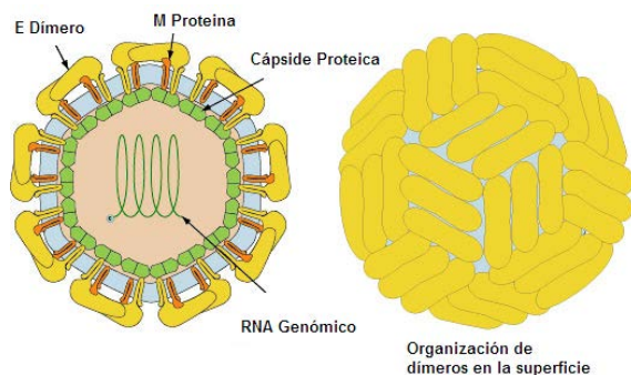
Figura 2. Cryo-EM. Estructura del virus del Zika [ZIKV].
