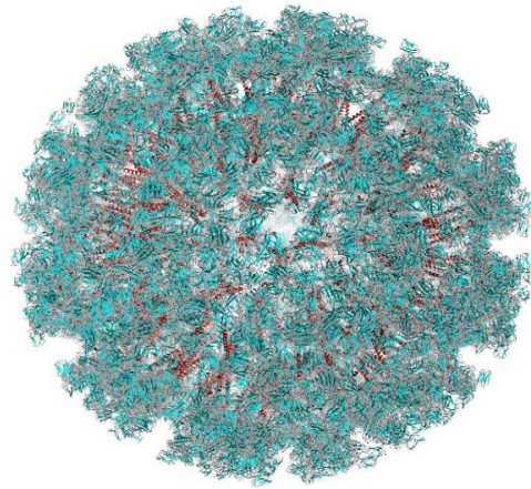
Figura 3. Estructura del virus Chikunguña.
