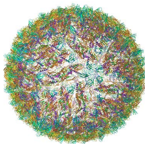
Figura 2. Cryo-EM. Estructura del virus del Zika [ZIKV].
