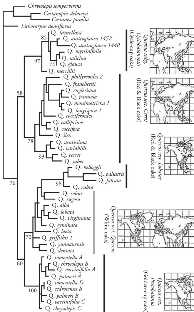
Fig. 1: arbre phylogénétique du genre Quercus obtenu par analyse de parcimonie des séquences ITS (Manos, 2001 ; adapté par Lepais, 2008).
