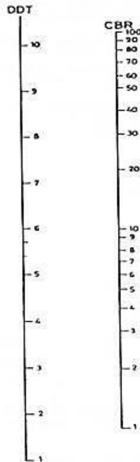
Gambar 2.2 Korelasi DDT dan CBR
