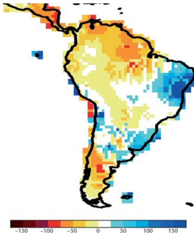
Figura 28. Mudanças previstas de vazões em porcentagem (%) na América do Sul, para o período 2061-2100, cenário A1B gerado pelo Modelo HadGEM1 (UK Met Office 2005).
