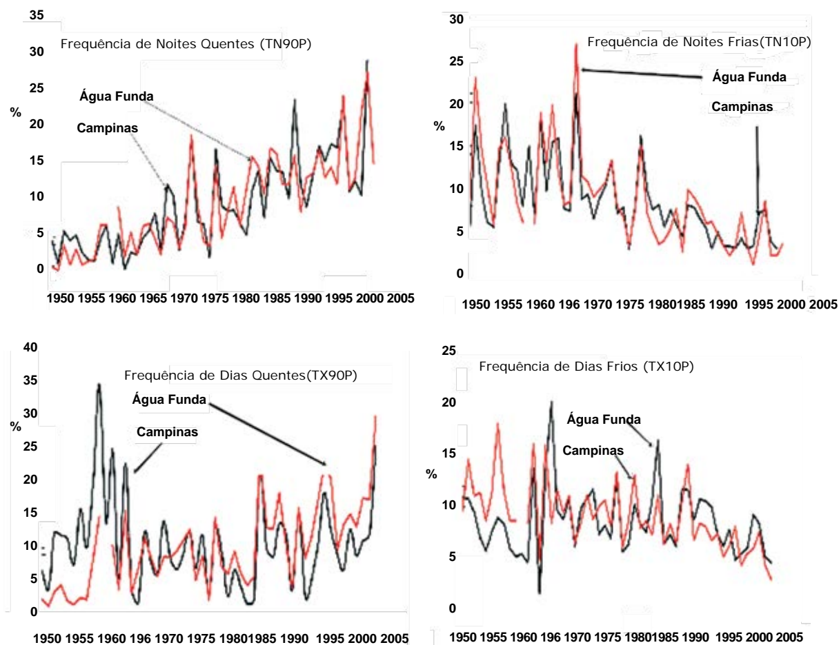
Figura 26. Tendências nas frequências (em %) de noites quentes (TN90P) e frias (TN10P), e de dias quentes (TX90P) e frios (TX10P) em Campinas e Água Funda, São Paulo. Índices são definidos em Vincent et al. (2005). (Fonte: T. Ambrizzi, IAG/USP).
