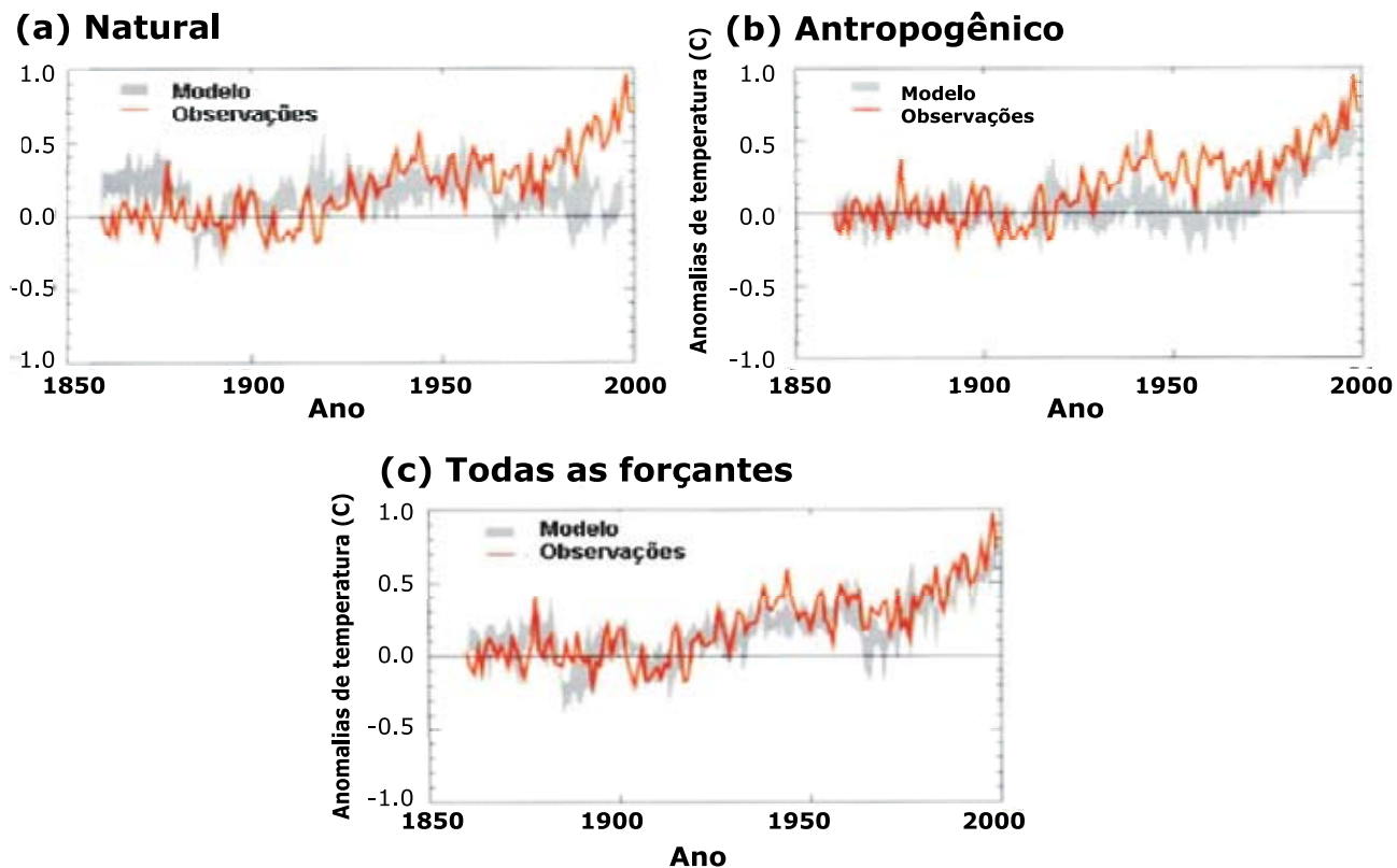
Figura 2. Anomalias globais de temperatura do ar relativas ao período 1850-1920, baseado em registros instrumentais, comparadas com a média de um conjunto de quatro simulações de modelos acoplados oceano-atmosfera forçados com: (a) forçamento solar e vulcânico somente, (b) forçamento antropogênico que inclui gases de efeito estufa, mudanças no ozônio troposférico e estratosférico e o efeito direto e indireto de aerossóis de sulfato, e (c) combinação de todas os forçamentos (naturais e antropogênicos). A linha vermelha representa as observações e a área em cinza representa os quatro modelos climáticos usados. As médias são anuais (Fonte: IPCC 2001a).
