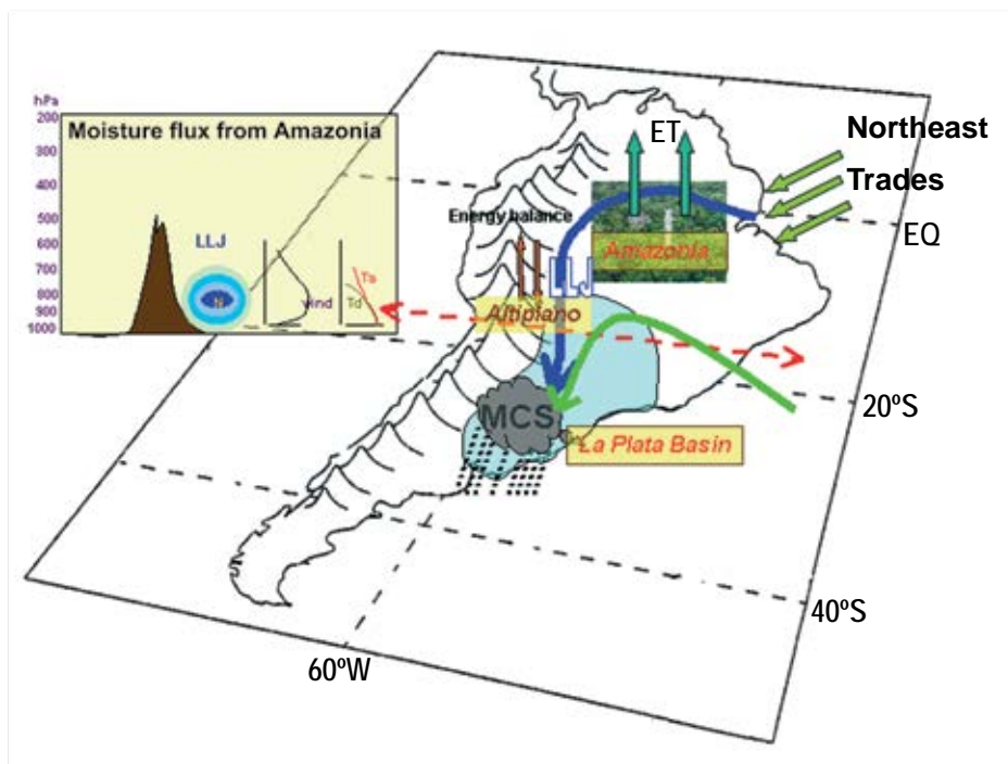
Figura 13. Modelo conceitual do jato de baixos níveis ao leste dos Andes que transporta umidade da Amazônia (flecha azul) e do oceano Atlântico subtropical (flecha verde) (Fonte: Marengo et al. 2004).
