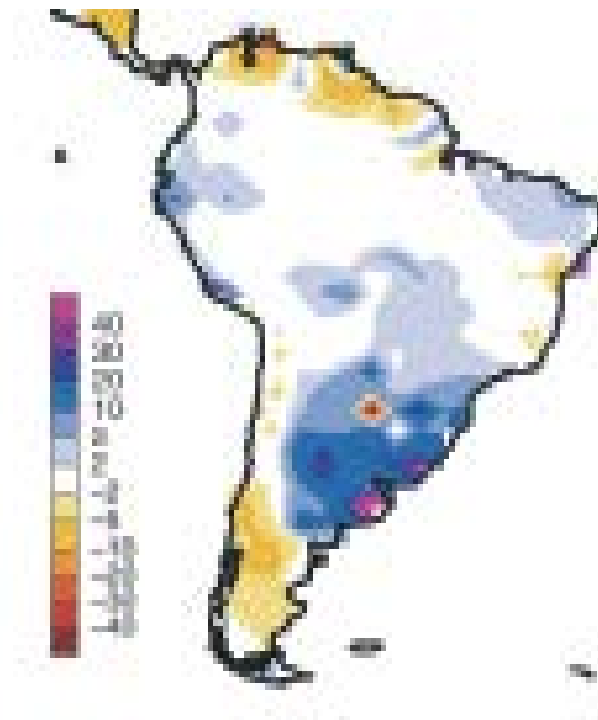
Figura 20. Mudança relativa de vazões durante o século XX na América do Sul. Valores são em porcentagem (%) para o período 1971-98 em relação ao 1900-70. Escala de cor aparece na esquerda da figura (Fonte: Milly et al. 2005)
