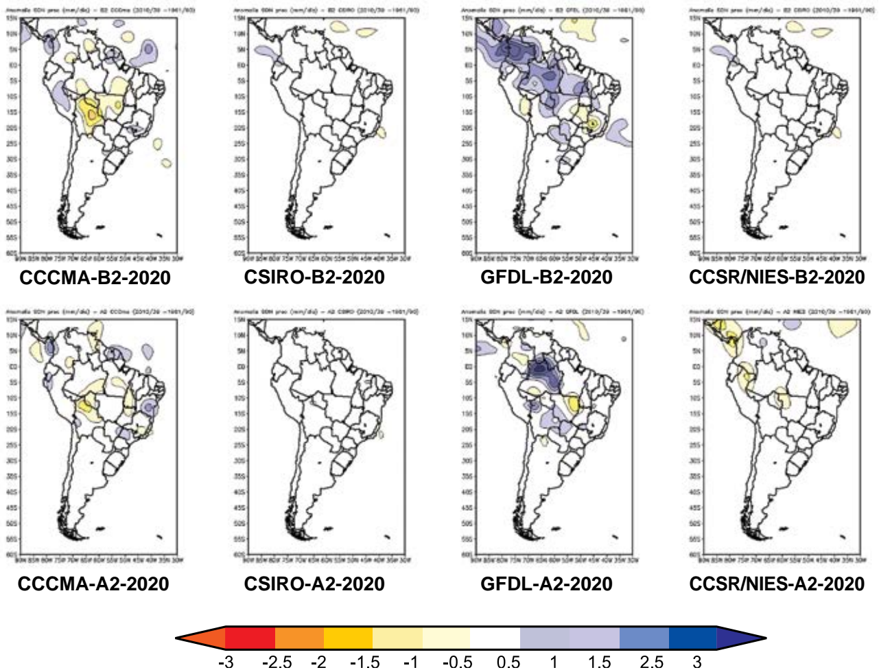
Figura 8. Projeções de anomalias de chuva para SON com referência ao período base 1961-90 para América do Sul. Os modelos são os CCCMA, CSIRO, GFDL e CCSR/NIES. Os cenários são A2 e B2 para time-slice centrado em 2020.
