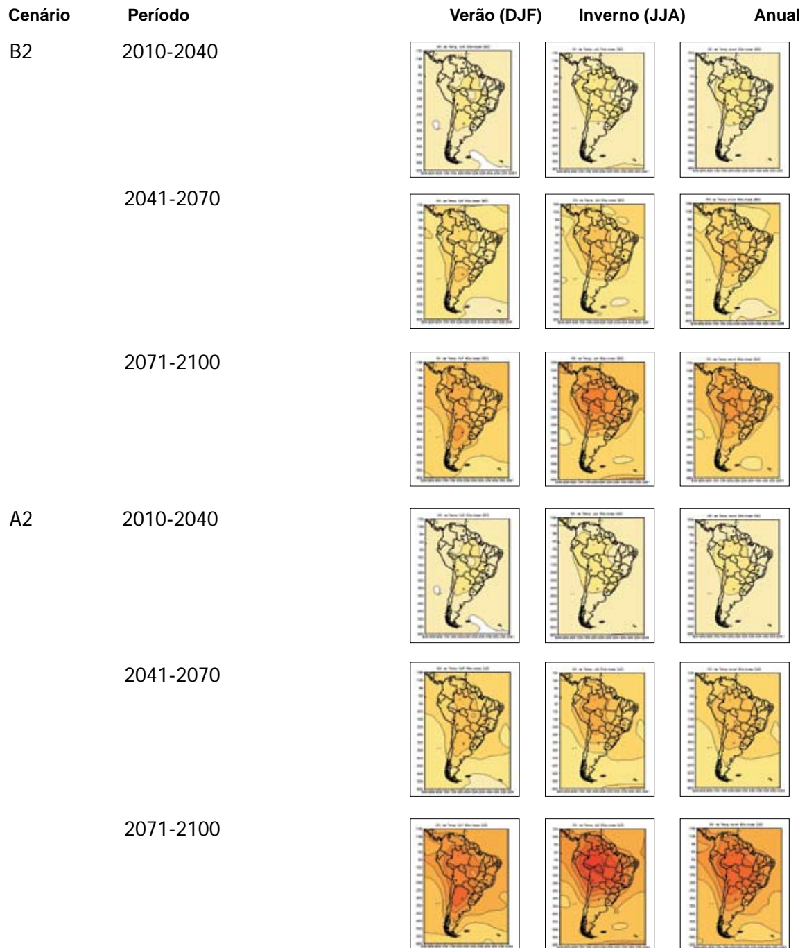
Figura 26. Média sazonal de verão (DJF), inverno (JJA) e anual dos cinco AGCMs para anomalias de temperatura do ar nos cenários A2 e B2, nos períodos 2010-2040, 2041-2070 e 2071-2100. As unidades estão em °C.
