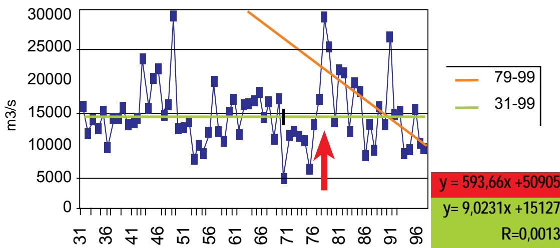
Figura 8. Vazões do rio São Francisco em Sobradinho durante dezembro-janeiro-fevereiro no período 1931-1998. A linha verde representa a tendência durante 1931-99 e a linha vermelha representa a tendência durante 1979-99. (Fonte: G. Sampaio, CPTEC/INPE).
