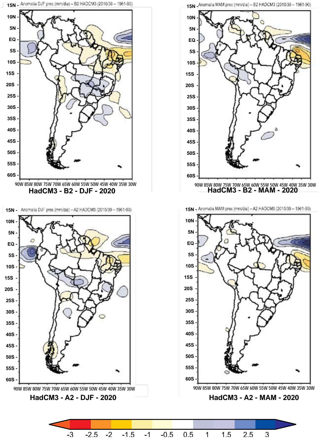
Figura 6. Projeções de anomalias de chuva para DJF e MAM com referência ao período base 1961-90 para América do Sul. Os cenários são A2 e B2 pelo modelo HadCM3. O time-slice é centrado em 2020.
