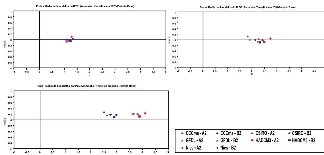
Figura 37. Diagrama de dispersão com anomalias anuais de temperatura (°C) e chuva para a bacia do Prata, nos time slices centrados em 2020 (painel superior), 2050 (painel médio) e 2080 (painel inferior) em relação ao clima atual 1961-90. Os diagramas foram elaborados considerando os cinco modelos globais de IPCC-TAR mostrados na parte inferior da Figura, para os cenários A2 (vermelho) e B2 (azul).
