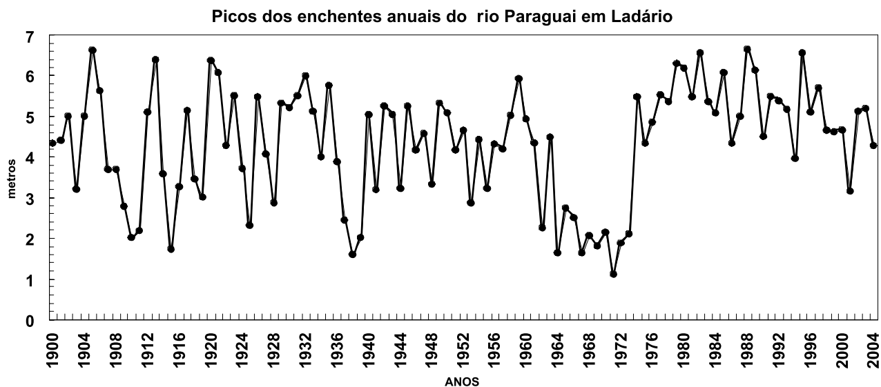
Figura 15. Níveis máximos do rio Paraguai em Ladário (Fonte: R. Clarke, IPH/UFRGS).
