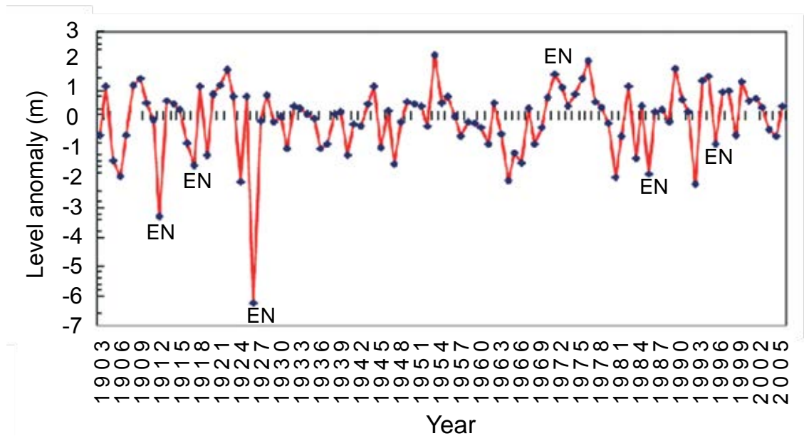
Figura 9. Nível médio do rio Negro em Manaus, AM desde 1903 até 2005. Valores na figura são anomalias em relação à média de 1903-2004. EN mostra a presença do ano El Niño .
