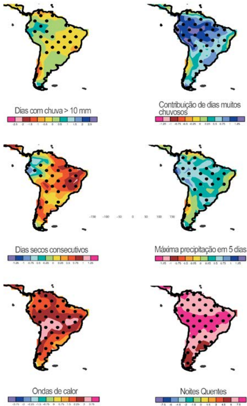
Figura 27. Compostos de mudanças em extremos climáticos de seis modelos do IPCC-AR4 para o cenário A1B, e apresentando diferenças entre o futuro (2080-2099) e o presente (1980-1999). Os índices de extremos são definidos no item 2.2: R10 - número de dias com chuva intensa acima de 10mm dia -1 , R95P- fração total de precipitação devido a eventos de chuva acima do percentual de 95th, CDD - dias secos consecutivos, RX5day - máxima precipitação acumulada em cinco dias, HWI - ondas de calor, TN90 - porcentagem de noites quentes. Valores gerados pelos modelos em cada ponto de grade foram normalizados em relação à média do modelo e depois o composto da média dos oito modelos foi calculada. Os pontos nos mapas correspondem a áreas, onde ao menos quatro dos seis modelos mostram mudanças estatisticamente significativas. (Fonte: Tebaldi et al. 2006).
