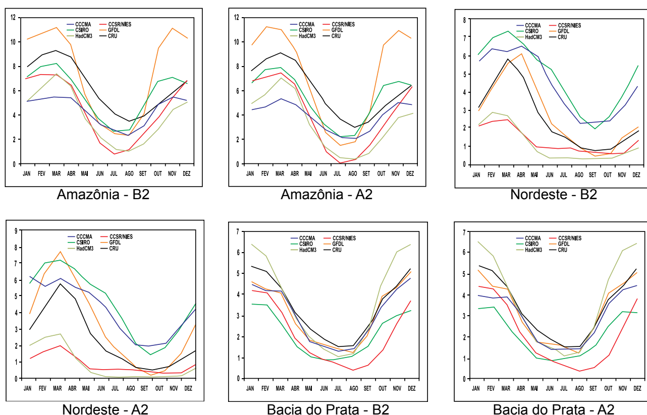
Figura 31. Variação sazonal de chuva em três regiões do Brasil (domínio na Figura 30) para o clima do presente (CRU) e para os futuros (2050-2100) cenários A2 e B2 dos modelos de IPCC: CCCMA, CSIRO, HadCM3, CCSR/NIES, GFDL. As unidades estão em mm dia -1 .
