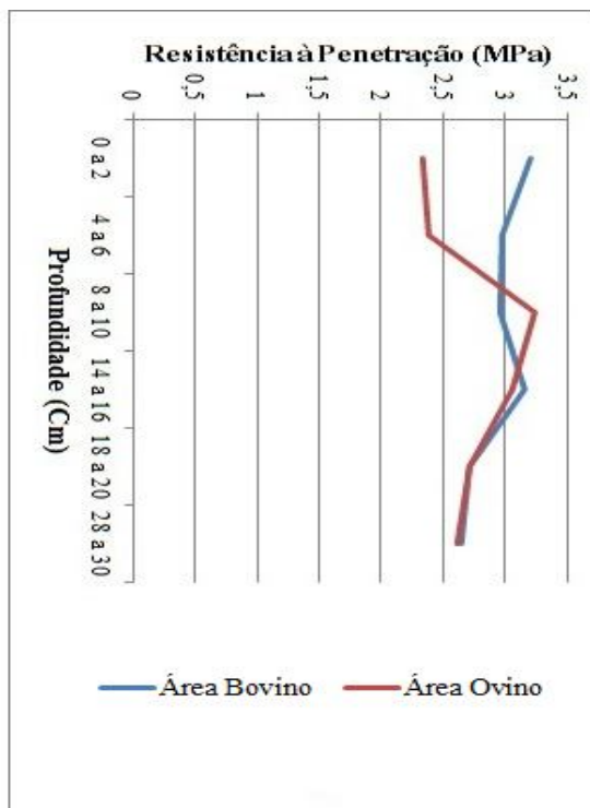
Figura 1. Resistência à penetração em função da profundidade do perfil do solo e comparação entre os sistemas de criação.
