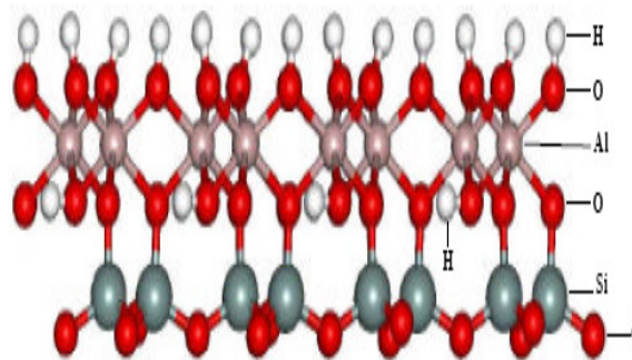
Figura 1 - Estrutura da caulinita (Adaptado de Castro, 2007).
