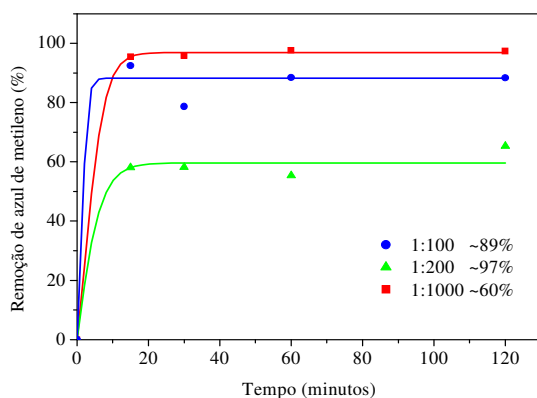
Figura 3 - Influência da quantidade de adsorvente na adsorção de azul de metileno em caulinita.
