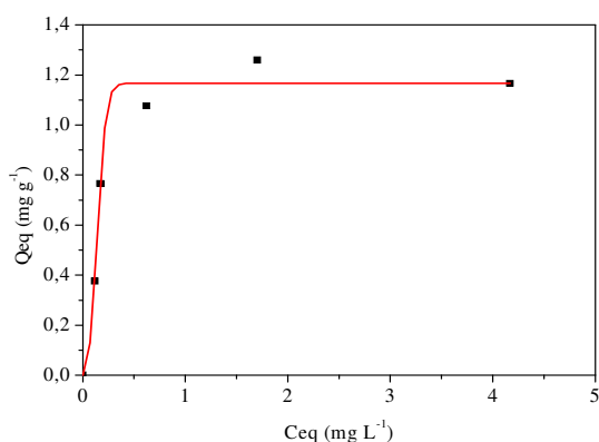
Figura 4 - Isoterma de adsorção de azul de metileno em caulinita rosa.
