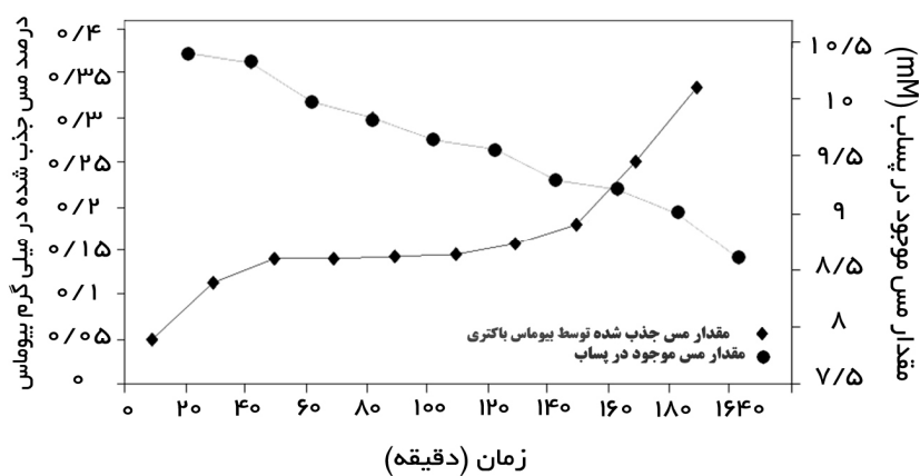
نمودار ۱: نتایج بررسی جذب اتمی باکتری لیز شده ایزوله ۱۳ پسدو مونااس از محیط کشت مایع حاوی فلزات سنگین مس
