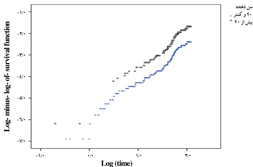
شکل ۲: بررسی فرض ثابت بودن نسبت مخاطره با استفاده از نمودار پراکنش \text{Log}(-\log(t)) بر روی \log(t) بر حسب سن دهنده
