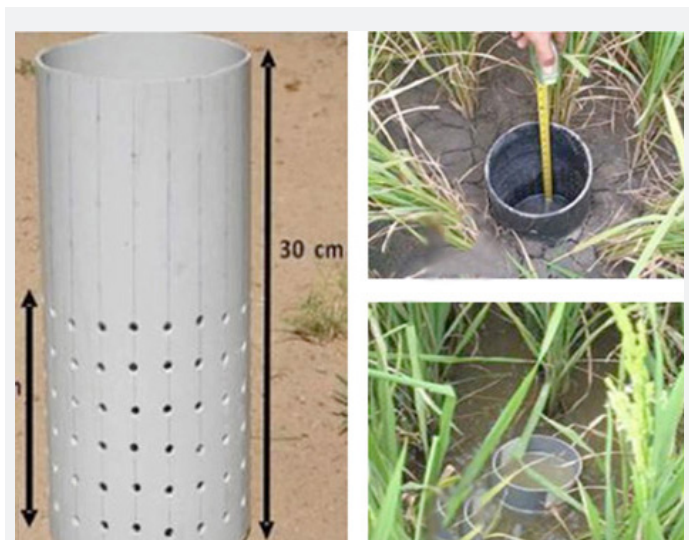
Picha Na.5.2. Kielelezo cha bomba la urefu wa sm 30 lililobolewa mpaka urefu wa sm 15cm (kushoto) likiwa limeshindiliwa kwenye udongo shambani kwa kina kinachotakiwa kabla ya kufurikisha maji (katikati) na baada ya kufurikisha (kulia). Picha na : Charles Chuwa /TARI Dakawa.
