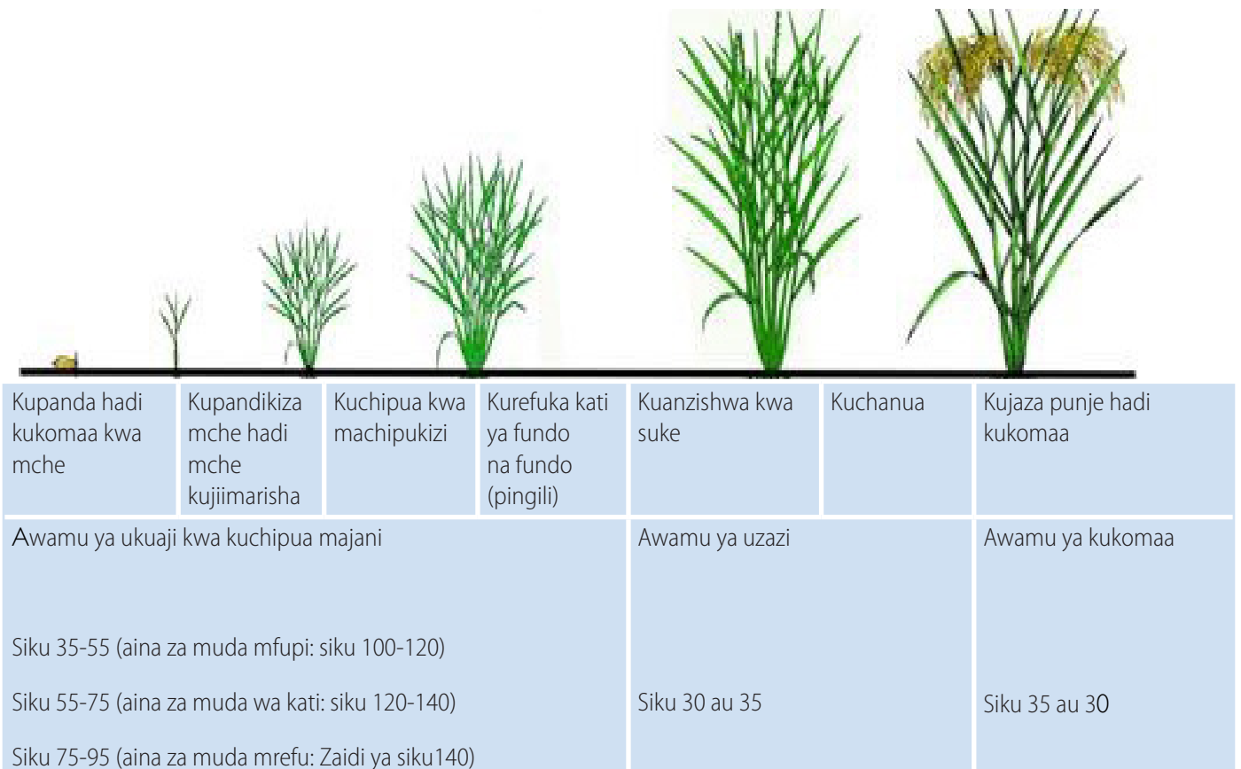
Picha Na. 5.1. Awamu na hatua za ukuaji mimea ya mpunga (Imenukuliwa kutoka IRRI).
