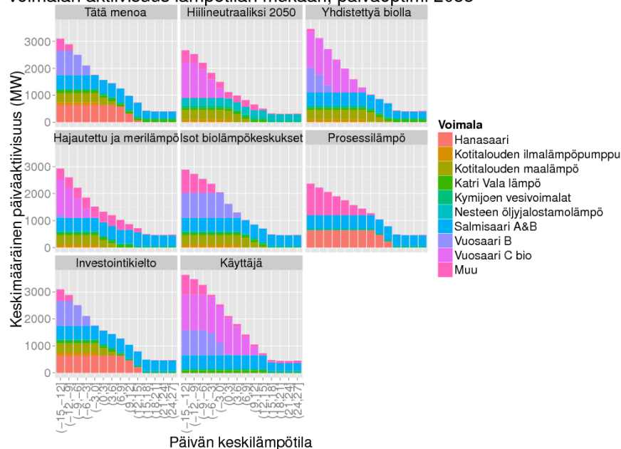
Kuva 5. Helsingin päivittäinen kaukolämpötase vuorokauden keskitenhona ilmoitettuna voimalaitoksittain. Tarve on eritelty päivän keskimääräisen ulkolämpötilan mukaan.
