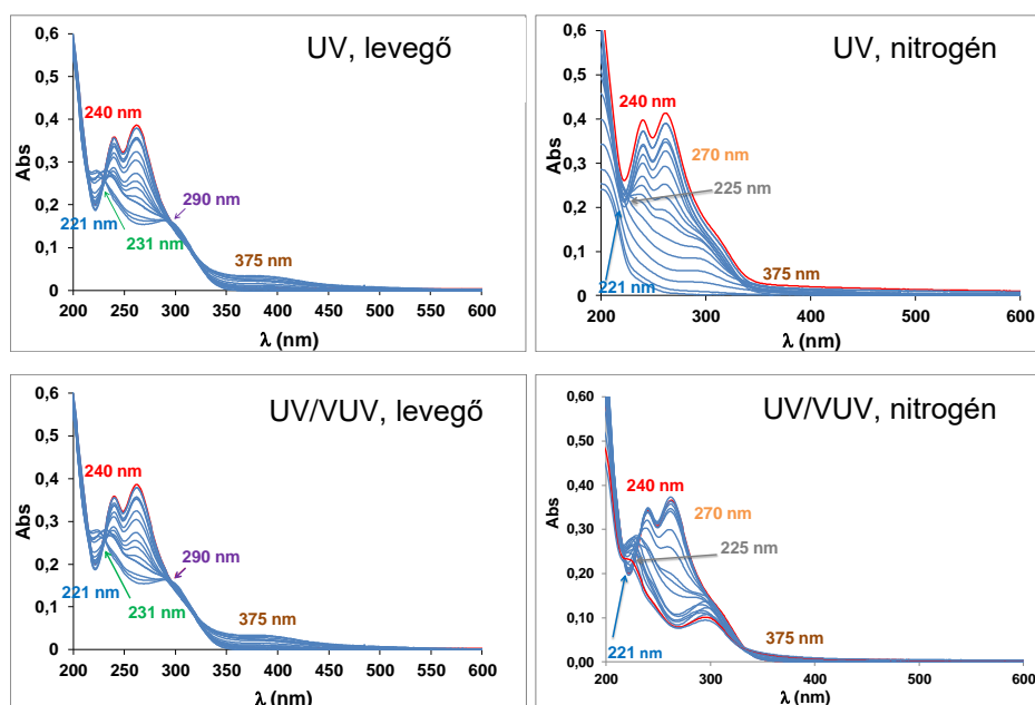
2. ábra Oldott oxigén hatása a spektrumokra UV és UV/VUV fotólízis során
