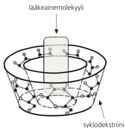
Kuva 1. Esimerkki syklodekstriinin sitoutumisesta lääkeaineeseen.
