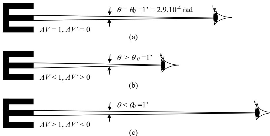
Figura 27. Angle de resolució (i agudeses visuals AV i AV' ). (a) Agudeses visual normal. (b) Agudeses visual per sota de la normal. (c) Agudeses visual per sobre de la normal.
