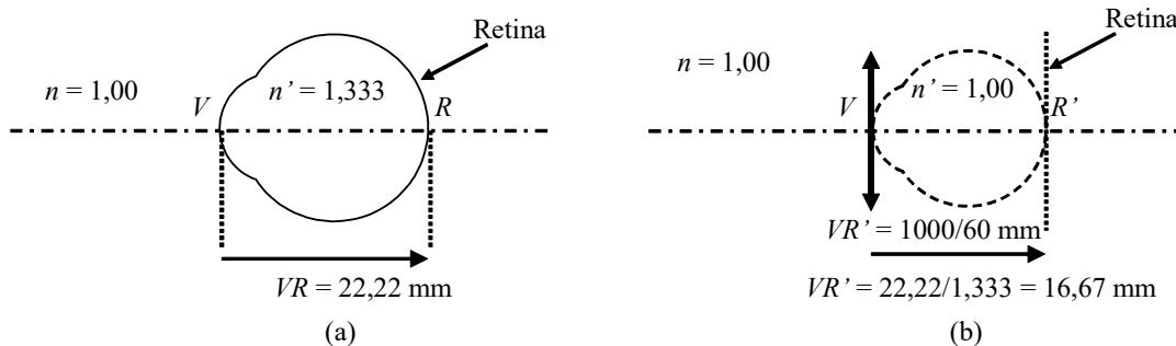
Figura 4. Esquema d'ull emmetrop reduït mitjançant: (a) Un dioptrè esfèric. (b) Una lent prima.
