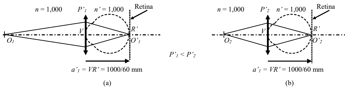
Figura 5. Esquema d'ull emmetrop reduït mitjançant: (a) Un dioptre esfèric. (b) Una lent prima.
