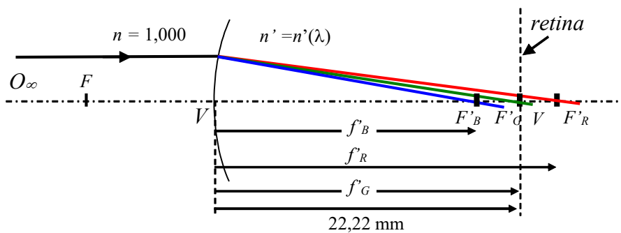
Figura 15. Ull emmetrop sense acomodar i dispersió cromàtica.
