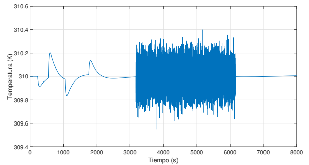
Figura 5: Perfil de temperatura en el sensor del modelo. Se simula un fallo en el sensor que introduce ruido entre el segundo 3240 y el segundo 6715.
