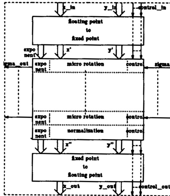
Figura 2.4: Arquitectura de FP CORDIC. Figura de de Lange et al. (1988)
