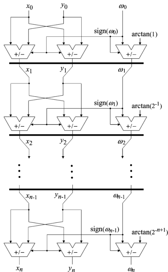
Figura 2.3: CORDIC convencional con pipelining . Extraído de Meher et al. (2009)
