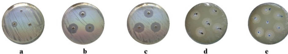
Gambar 2. Diameter zona hambat radi 20 (termasuk diameter sumuran 6 mm) terhadap S. aureus dari cairan kultur hari ke 1-3 (a), 4-6 (b), 7-9 (c), 10-14 (d) dan 15-20 (e).
