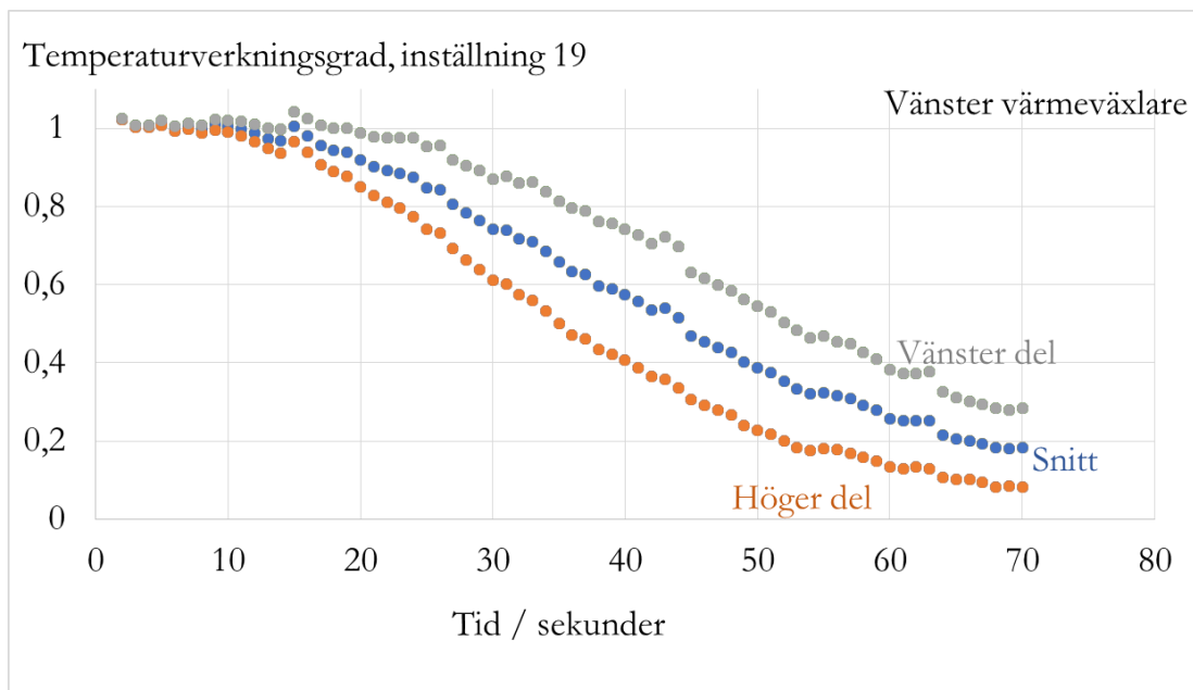
Figur 16. Temperaturverkningsgrad för vänstra samt högra halvan av den vänstra värmepumpen. I blått visas snittet av de båda halvorna.
