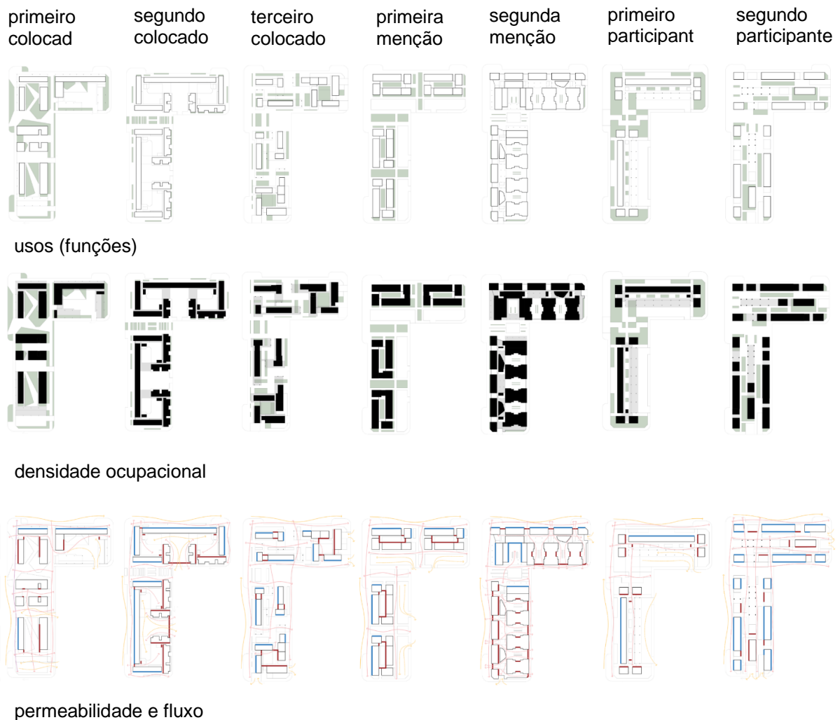
FIG.03: Matriz comparativa.
