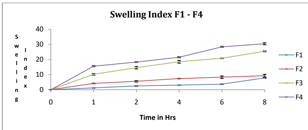
Fig. 3: Swelling Index of formulation F1 - F4
