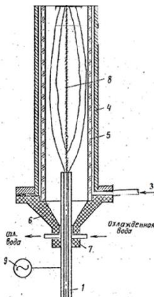
Рисунок 3.1.1 – Экспериментальная установка:
