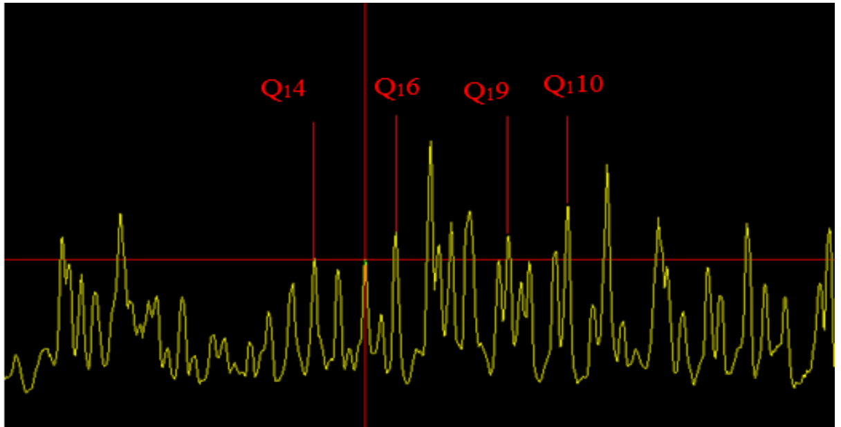
Рисунок 2.2.5 – Спектр полос гидроксила в плазме аргон – воздух с 30% содержанием воздуха
