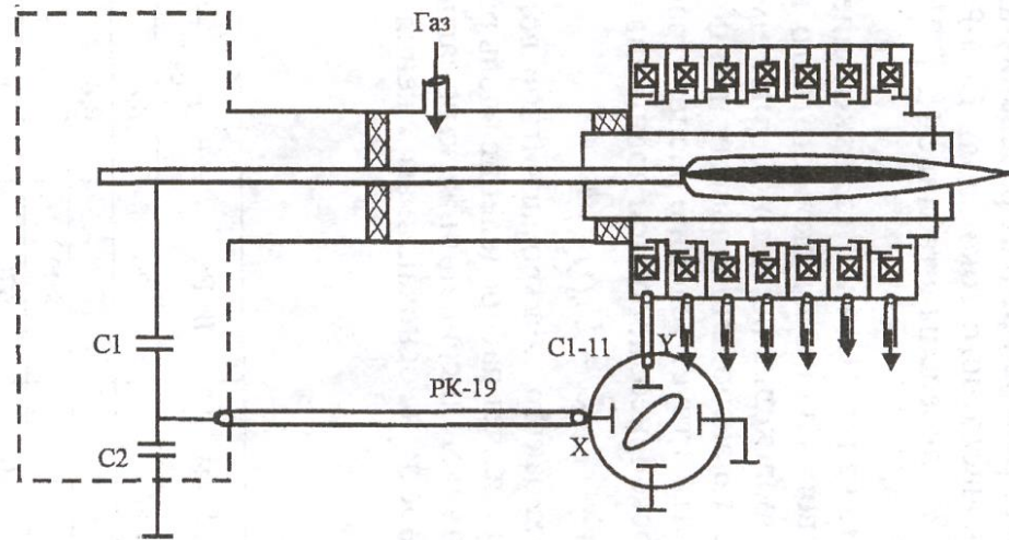
Рисунок 1.12 – Схема экспериментальной установки
