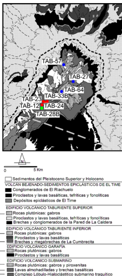
Fig. 2. - Mapa geológico de la Caldera de Taburiente (Colmenero et al., 2012). Fig. 2.- Geological map of the Caldera de Taburiente (Colmenero et al., 2012).
