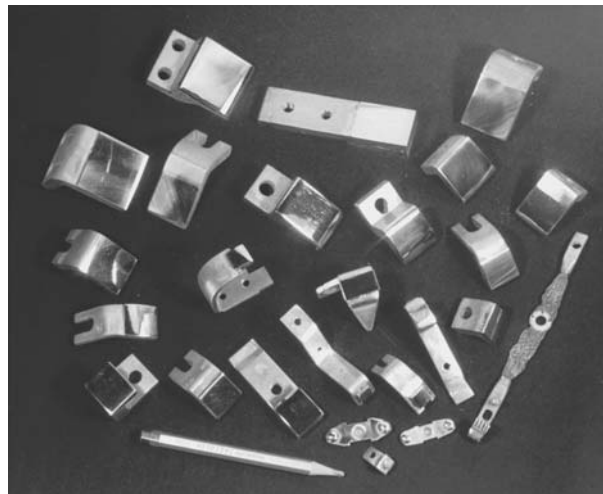
Figure 3. General view of contacts made with application of composite materials for electrical contacts Slika 3. Pogled na kontakte prigotovljene s rabljenjem kompozitno elektrokontaktne materijala
