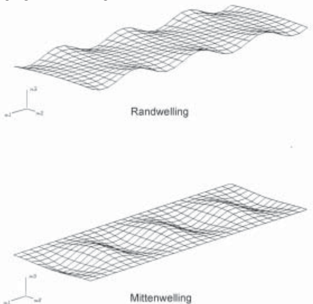
Bild 6. Mitten und randwelliges Blech Slika 6. Valovitost na sredini i na rubovima lima
