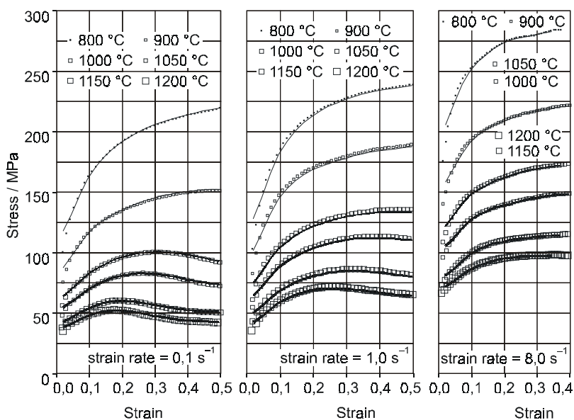
Figure 4. Hot flow curves for tool steel - experimental and predicted results, using a constant smoothing parameter ( w = 0,035 ) Slika 4. Krivulje zatezanja u vrućem za alatni čelik - eksperimentalni i predmnijevani rezultati upotrebom stalnog parametra glatkoće ( w = 0,035 )
