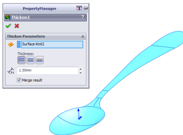
Slika 8. Opcija Thicken
