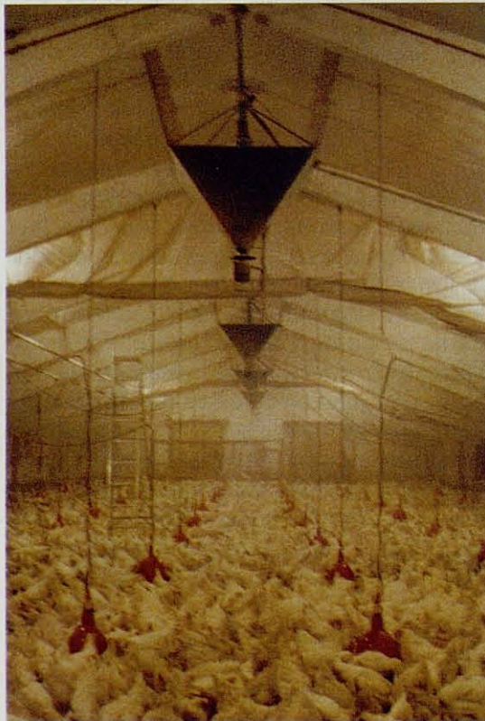
Las tolvas aspersoras, montadas en una nave a media crianza.
