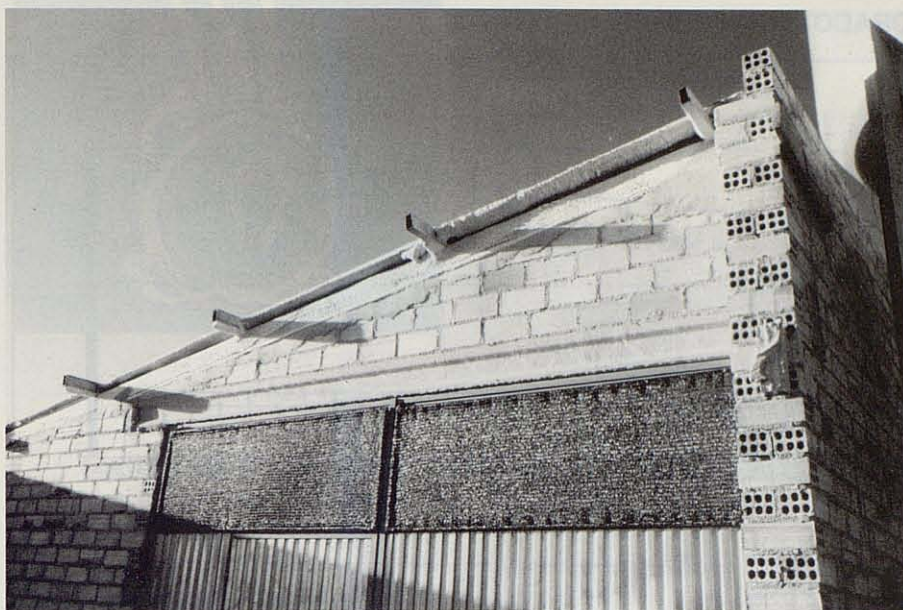
Los tabiques interiores sirven de apoyo a los correos. Es frecuente utilizar como aislante POLIURETANO proyectado. Se aplica interiormente una vez acabada la edificación. (Foto tomada en La Milla del Río (León)).
