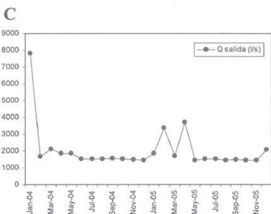
Figura 3. A.- Variación del volumen embalsado ( hm^3 ) en el embalse del Añarbe (enero 2004-diciembre 2005). B.- Caudal de entrada ( Q , l/s). C.- Caudal de salida mensual ( Q , l/s). A.- Variation of the dammed volume ( hm^3 ) in the Añarbe reservoir (January 2004-December 2005). B.- Entry volume ( Q , l/s). C.- Monthly exit volume ( Q , l/s).
