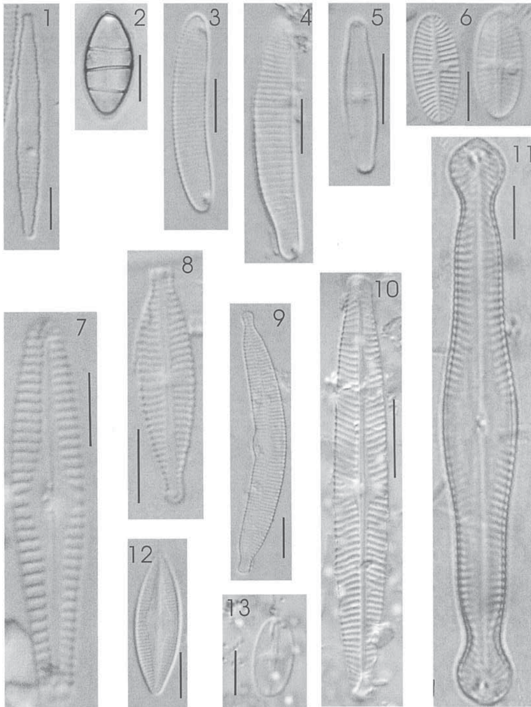
Figura 2. 1. Fragilaria capucina , 2. Diatoma mesodon , 3. Eunotia intermedia , 4. Eunotia minor , 5. Achnanthisidium minutissimum , 6. Planothidium distinctum , 7. Gomphonema rhombicum , 8. G. parvulum , 9. Hannaea arcus , 10. Navicula angusta , 11. Pinnularia polyonca , 12. Nupela lapidosa , 13. Psammothidium cf. subatomoides . Escala: 6 \mu\text{m} . 1. Fragilaria capucina , 2. Diatoma mesodon , 3. Eunotia intermedia , 4. Eunotia minor , 5. Achnanthisidium minutissimum , 6. Planothidium distinctum , 7. Gomphonema rhombicum , 8. G. parvulum , 9. Hannaea arcus , 10. Navicula angusta , 11. Pinnularia polyonca , 12. Nupela lapidosa , 13. Psammothidium cf. subatomoides . scale: 6 \mu\text{m}
