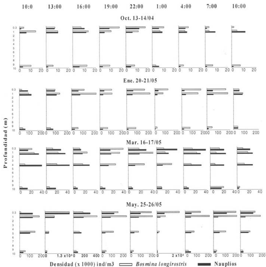
Figura 3. Lago Acuarela. Distribución vertical de Bosmina longirostris y nauplios. Lago Acuarela. Vertical distribution of Bosmina longirostris and nauplios.
