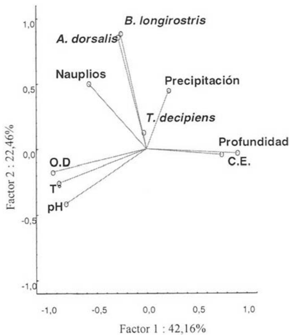
Figura 5. Lago Acuarela. Análisis de componentes principales para el zooplancton y las variables abióticas en los cuatro ciclos de muestreo. Lago Acuarela. Analysis of principal components for the zooplankton and the abiotic variables in the four sampling cycles.
