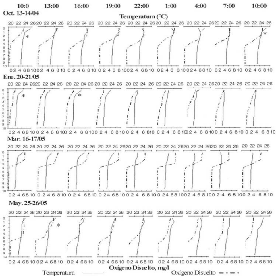
Figura 2. Lago Acuarela. Perfiles verticales de temperatura del agua y oxígeno disuelto para para las fechas de muestreo. * Estratificación térmica. Lago Acuarela. Vertical profiles of water temperature and dissolved oxygen for the sampling dates. * Thermal stratification.
