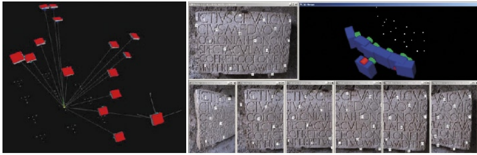
Fig. 8 – (a) Configurazione geometrica ottimale per calibrare una fotocamera digitale e determinarne i parametri di orientamento interno, utilizzando immagini convergenti a distanze diverse da un oggetto tridimensionale. (b) Tipica configurazione di immagini acquisite per modellare in 3D un oggetto misurando alcuni punti omologhi tra le immagini per ricavarne l'orientamento esterno.
