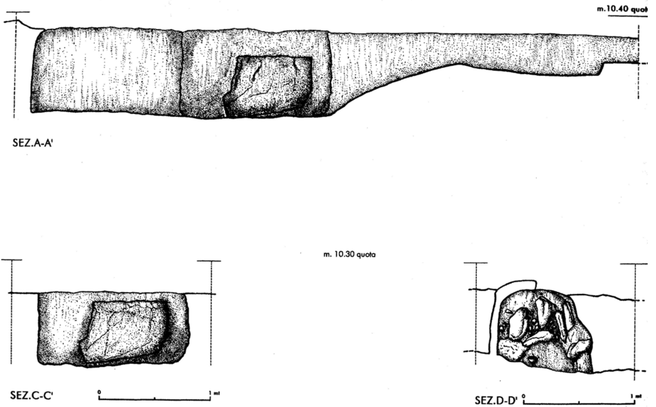
Fig. 4. Pescia Romana. Sezioni.
