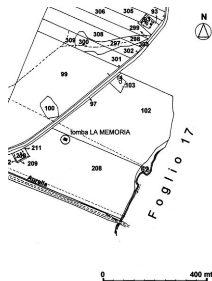
Fig. 2. Pescia Romana. Posizionamento della tomba (su foglio catastale 1:4.000).
