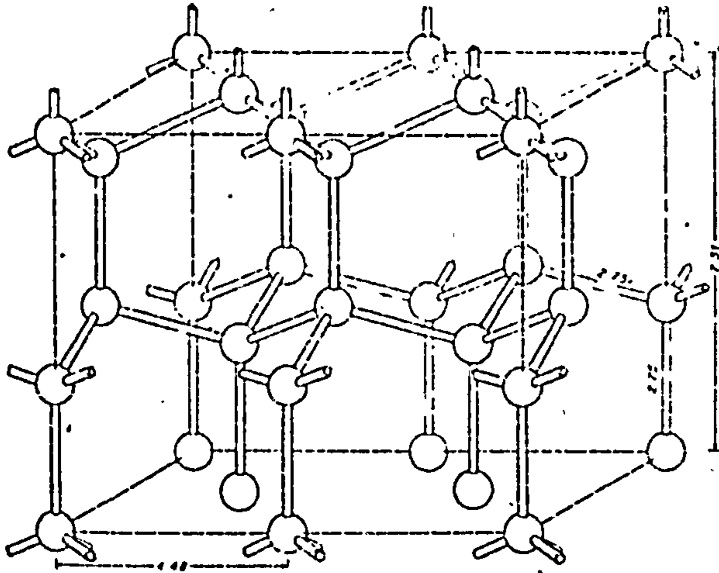
a) Ice I
