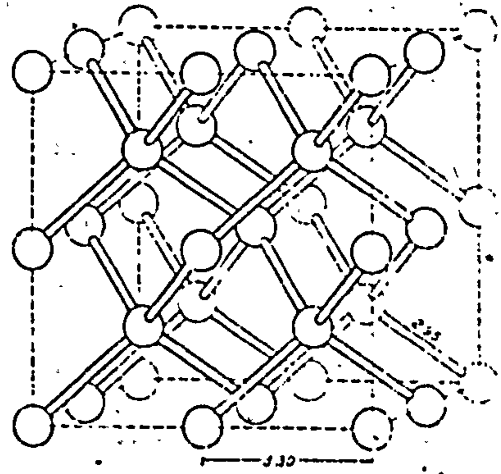
f) Ice VII
