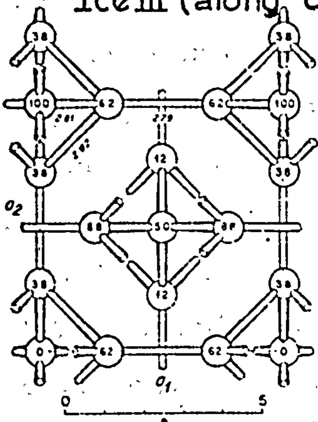
e) Ice VI (along c axis)
