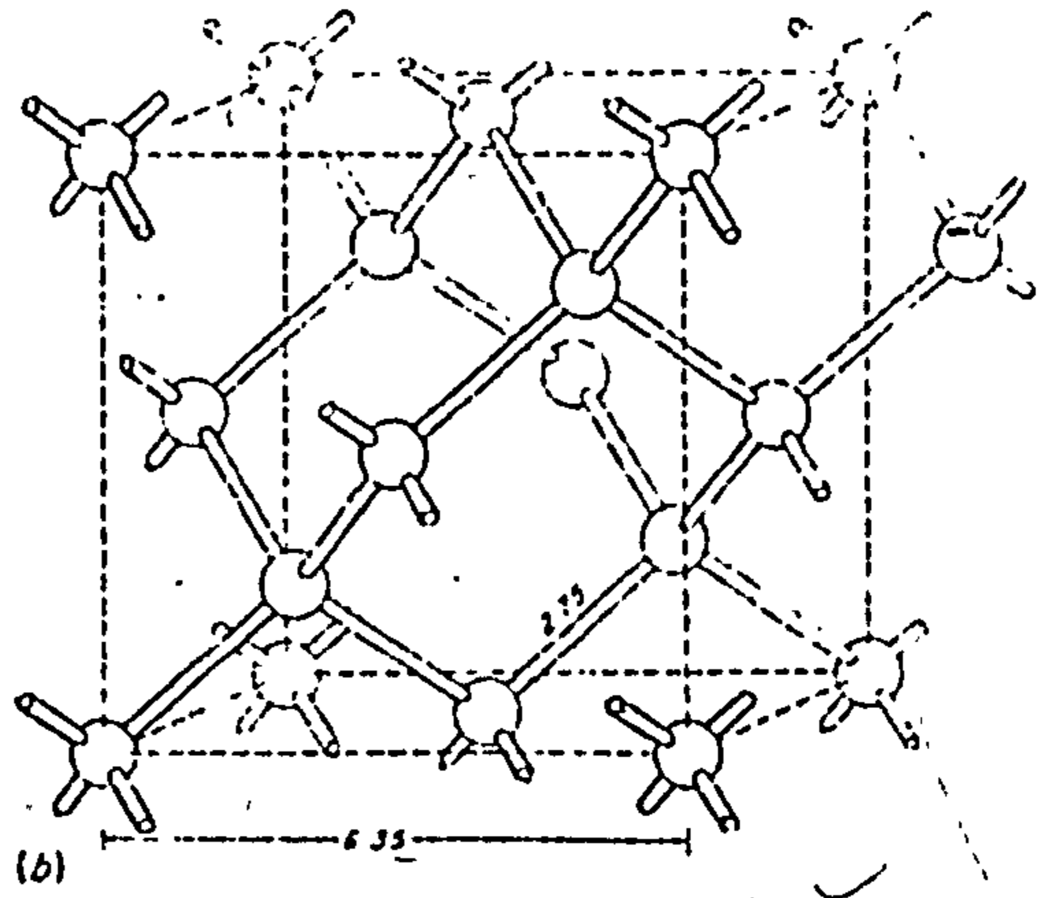
b) Ice Ic
