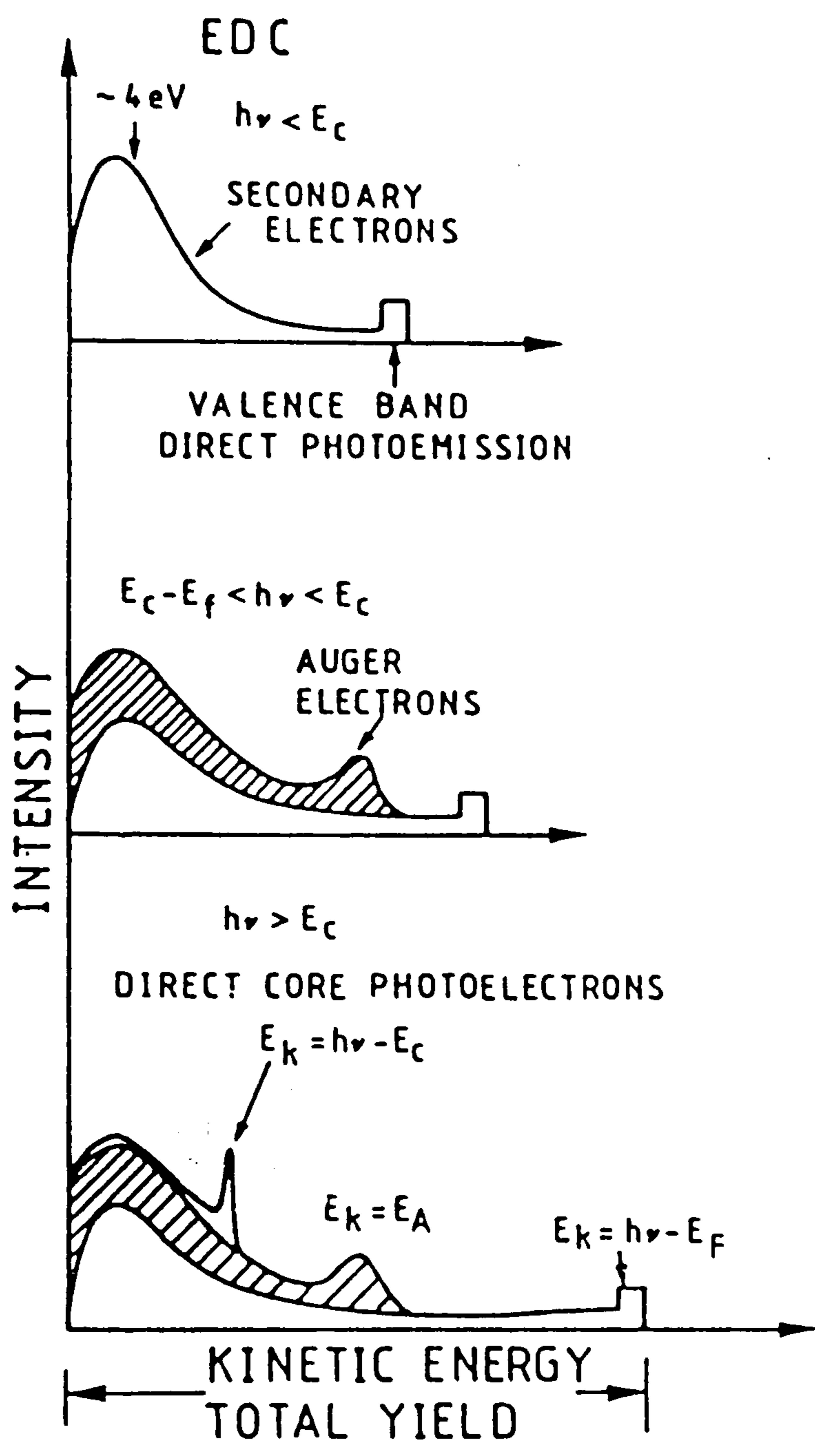
Fig. 1.1.12 Partial yield method (Davoli et al., 1988).
