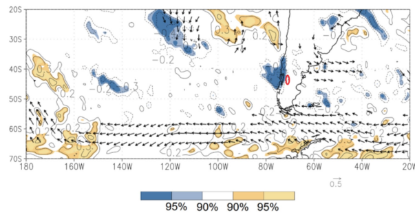
b) Vector y Divergencia de FVHI, DEFMAM
