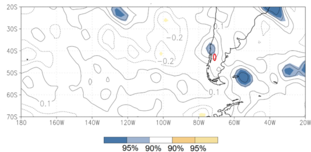
d) CMAP Precipitación, DEFMAM
