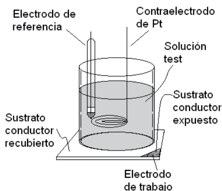
Figura 1: Celda electroquímica.
