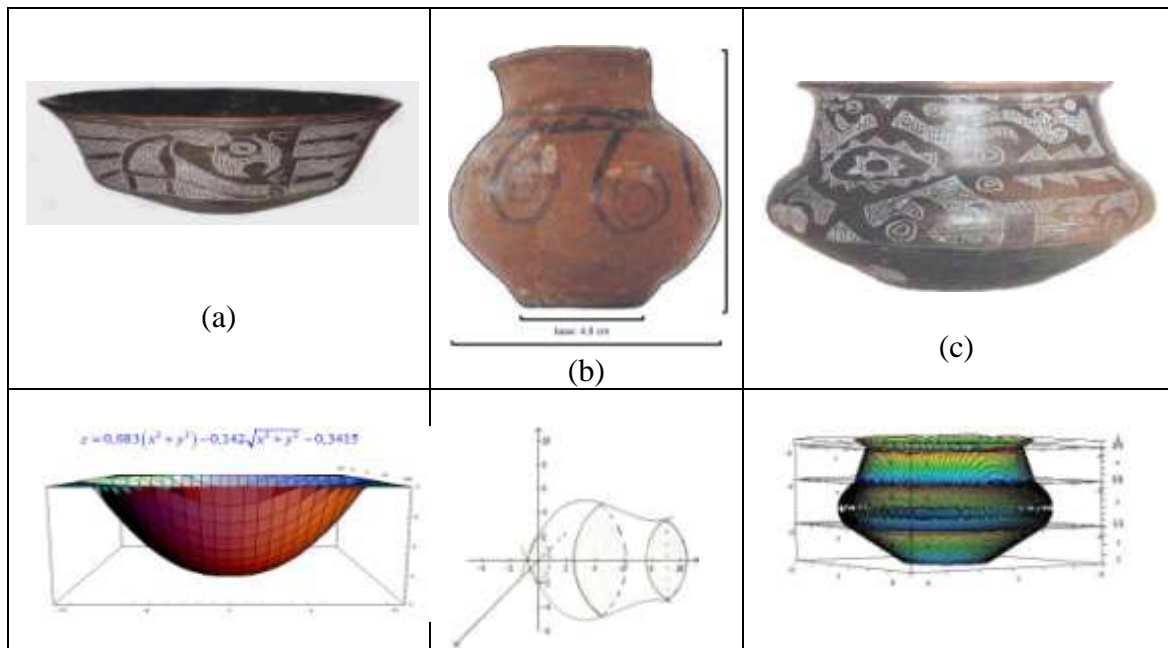
Figura 1: Vasijas escogidas para dicho estudio: (a) Modelo geométrico obtenido de la vasija tipo fuente realizada con rotación sobre el eje vertical, (b) Modelo geométrico de la vasija tipo cántaro girada y rotada sobre eje horizontal, y (c) Modelo geométrico de la vasija tipo cántaro de boca ancha obtenida sobre el eje vertical pero por partes, resultando con cuatro asignaciones
