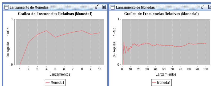
Fig. 4: Gráfica de frecuencia relativa de águilas vs. cantidad de lanzamientos de una moneda
