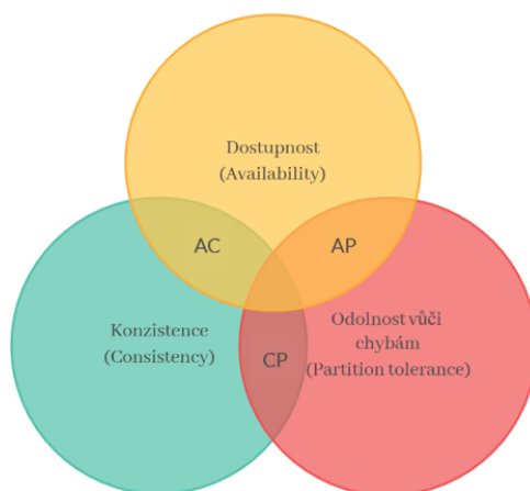
Obrázek 1: CAP teorém
