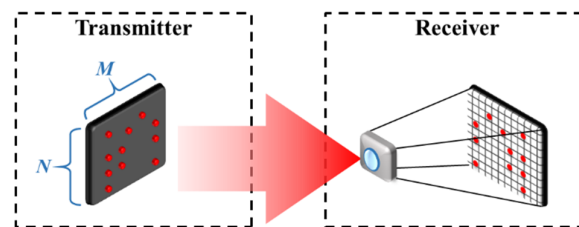
Figure 26. A visual MIMO scheme.
