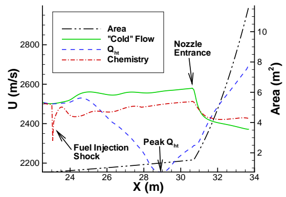
(d) u-Velocity
