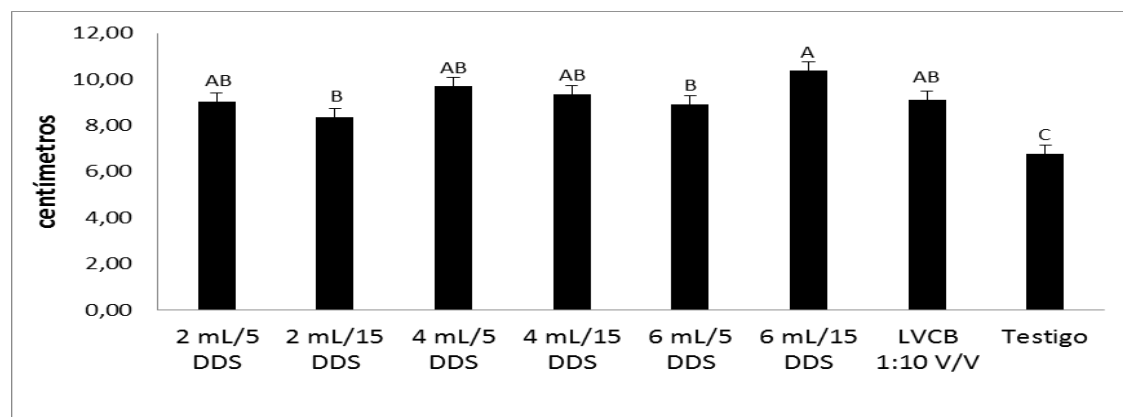
Figura 1: Valores medios de longitud (cm) de raíz a las aplicaciones de Trichoderma sp. y lixiviado de vermicompost bovino (LVCB). Los valores medios con letras diferentes difieren significativamente acorde a la prueba de Duncan ( p < 0,05 )
