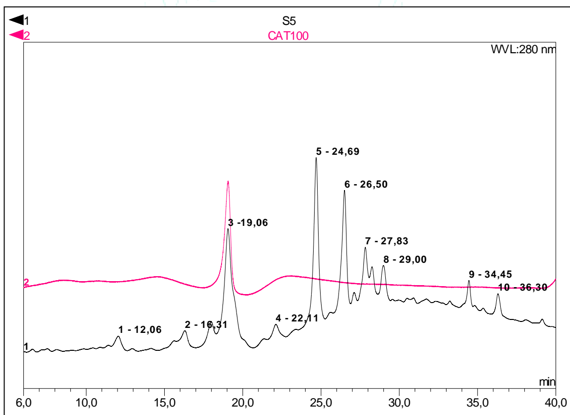
Fig. 5 : Chromatogrammes HPLC-DAD de la SF5 (1) et de la catéchine (2)
