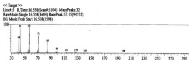
Gambar 1. Spektrum masa senyawa dengan waktu retensi 16,560 menit
