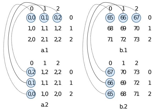
Gambar 1. Rotasi CCW pada larik: (a) koordinat larik, (b) elemen larik
