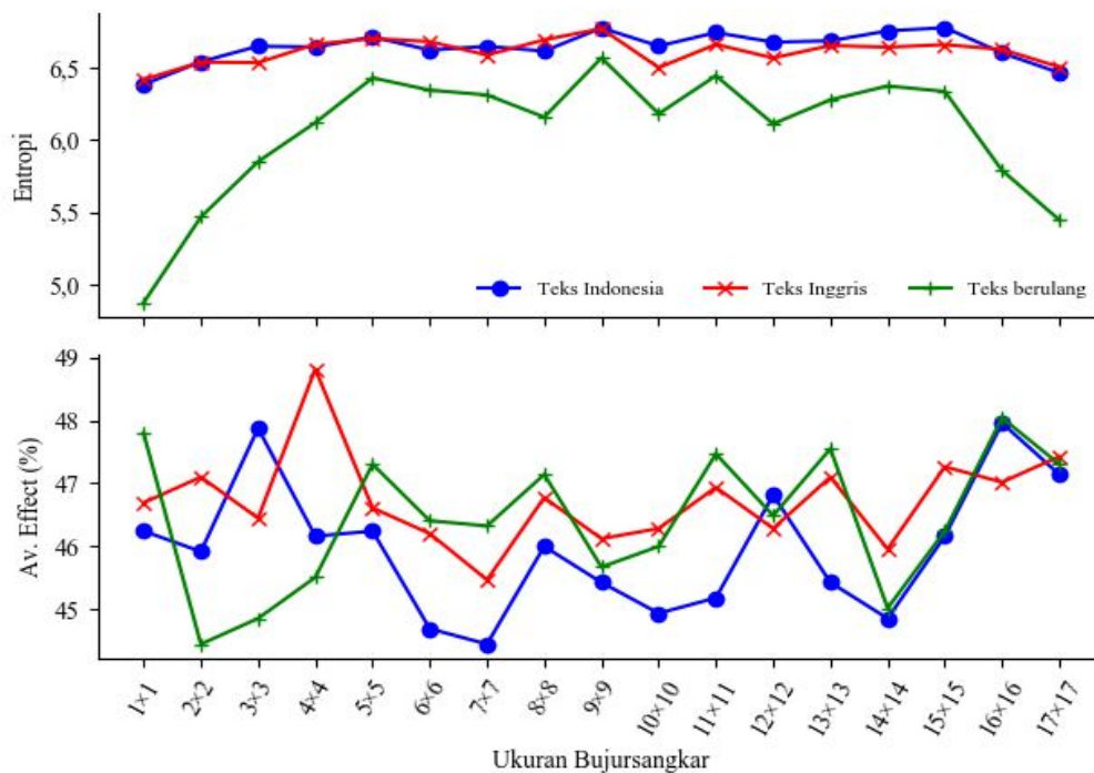
Gambar 4. Entropi dan AE sesuai ukuran bujursangkar
