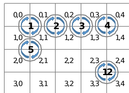
Gambar 3. Urutan rotasi bujursangkar 2 \times 2 pada larik 4 \times 5
