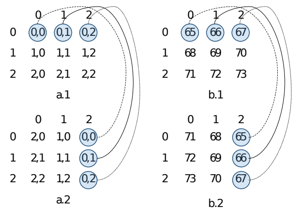
Gambar 2. Rotasi CW pada larik: (a) koordinat larik, (b) elemen larik
