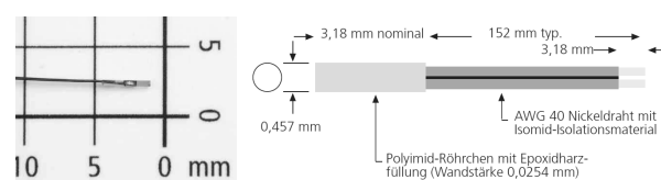
Fig. 1. Thermistor NTC 2K7MCD1.
