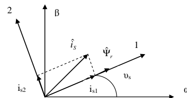
Fig. 2. Vector diagram of the IM state variables
