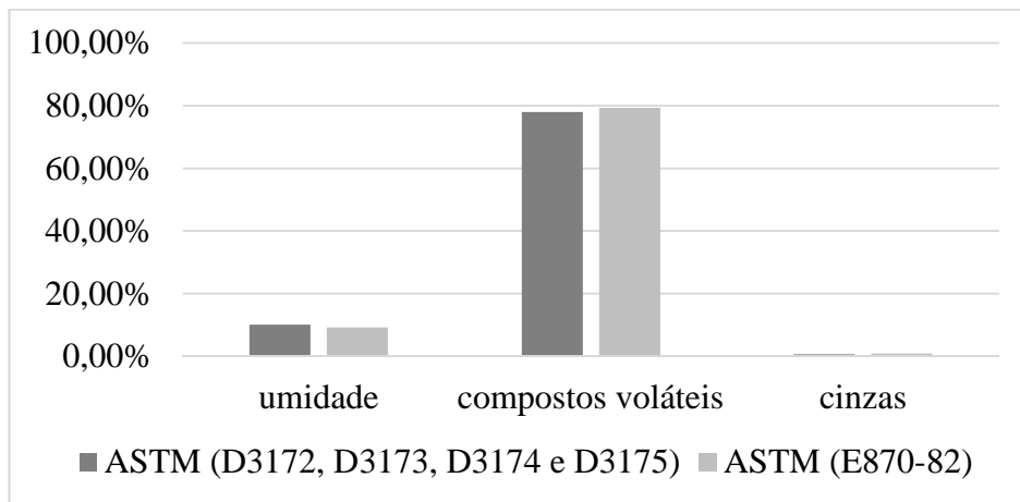
Figura 1: Comparação entre as Análises Imediatas ASTM (D3172, D3173, D3174 e D3175 ) e ASTM (E870-82)
